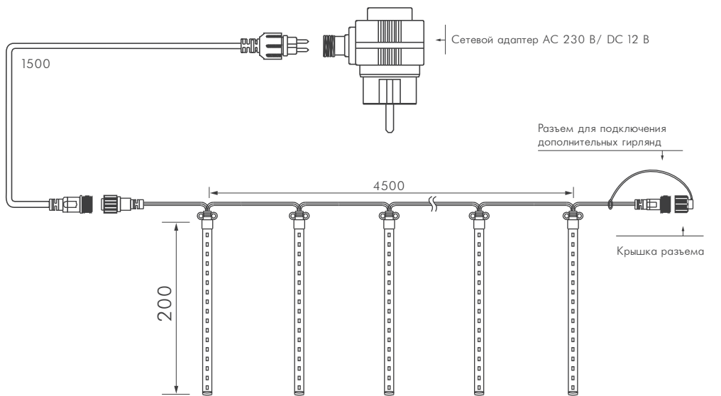
Рисунок 1. Схема подключения.
