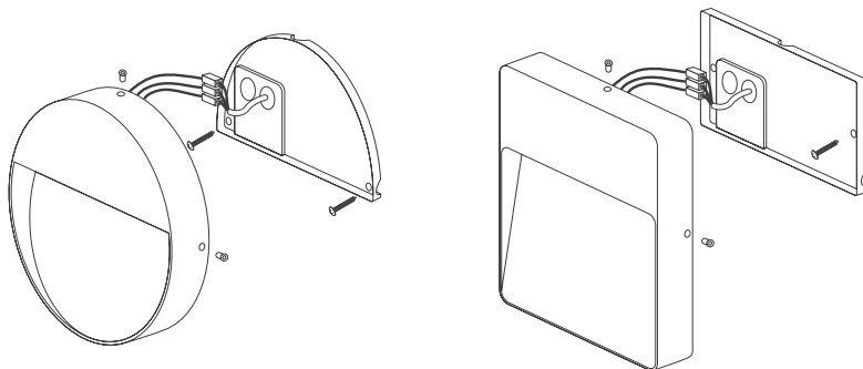
Рис. 2. Установка и подключение светильника
